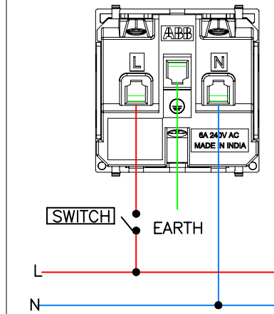
3+2 Pin socket
